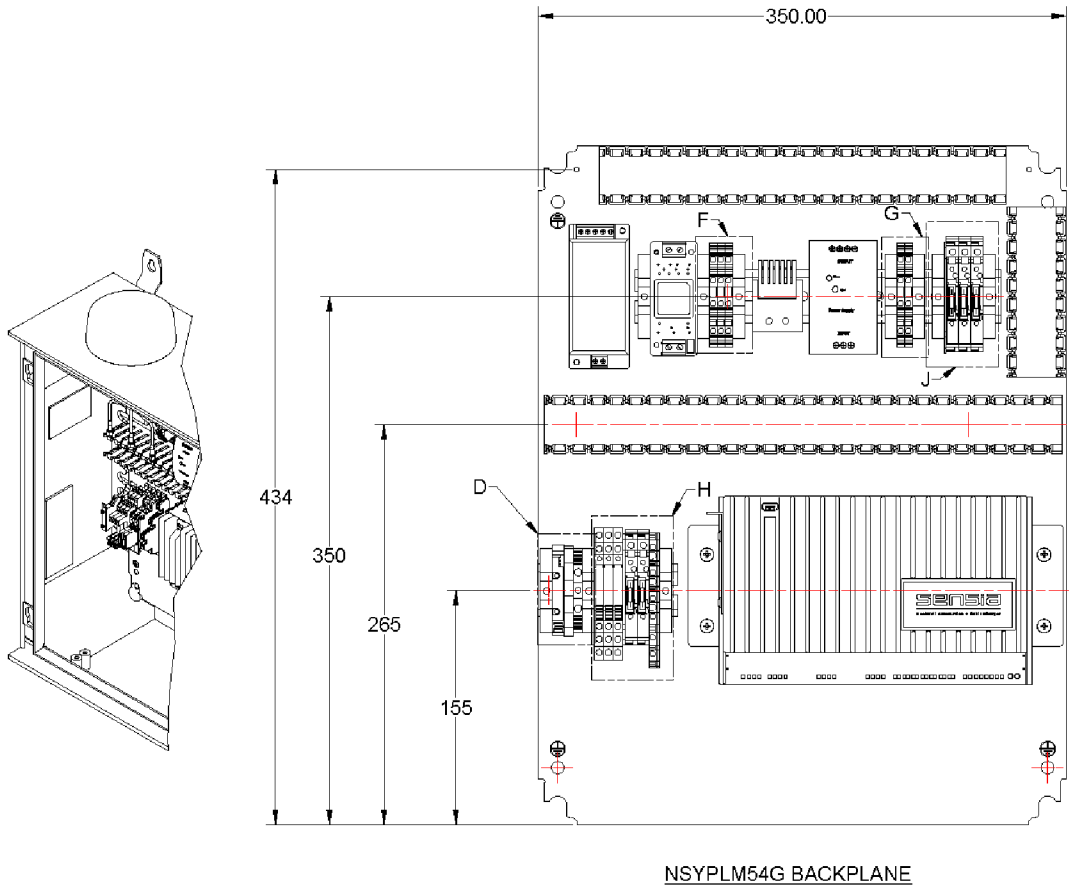
NSYPLM54G BACKPLANE
